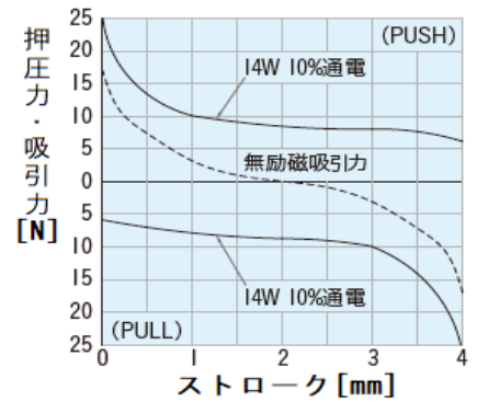
押圧力・吸引力特性
