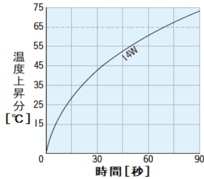
温度上昇特性
