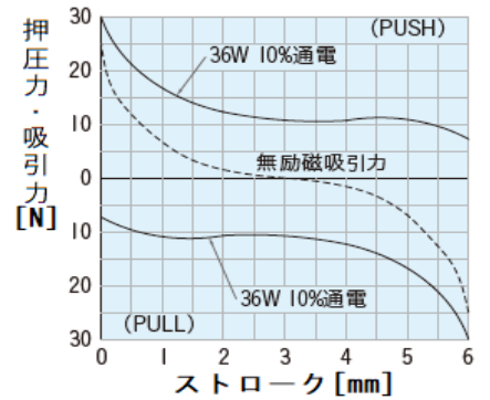
押圧力・吸引力特性
