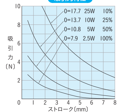
吸引力特性
