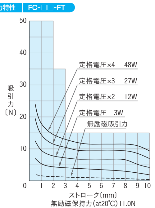
吸引力特性
