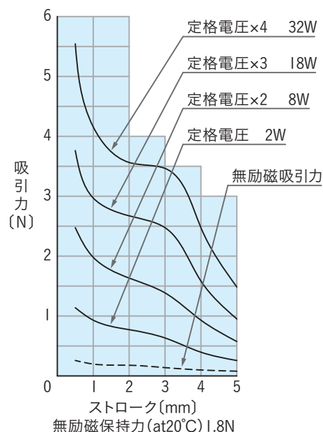
吸引力特性
