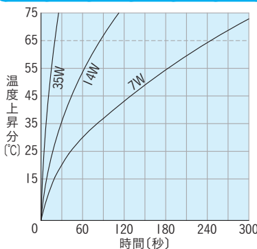
温度上昇特性 CA-154804 / CA-154808
