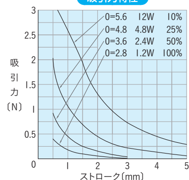
吸引力特性
