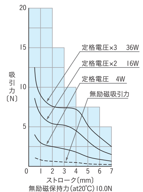
吸引力特性
