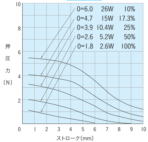
吸引力特性
