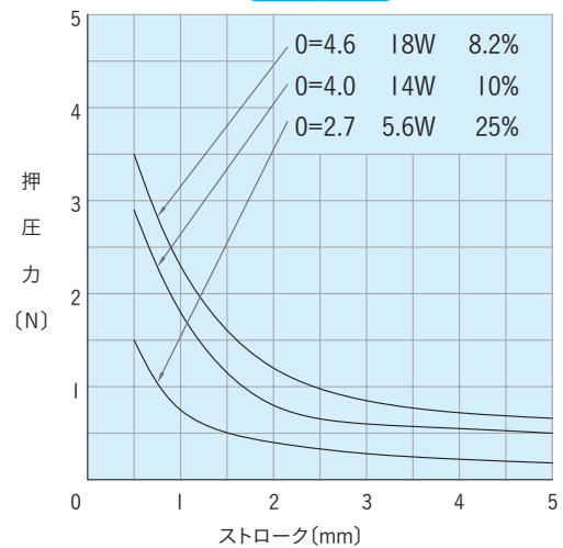
吸引力特性
