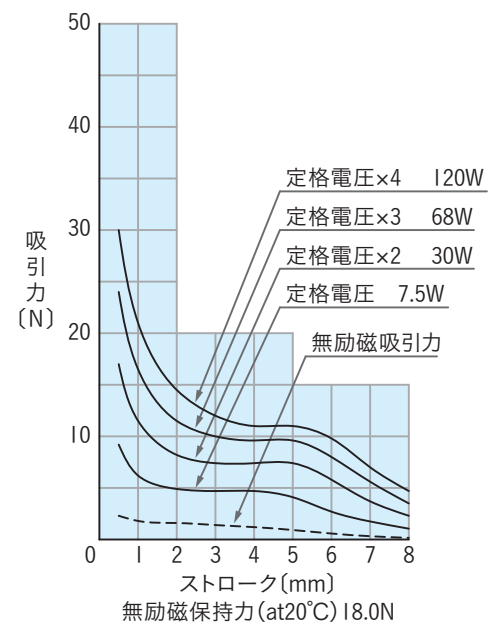
吸引力特性
