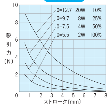
吸引力特性
