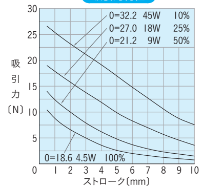
吸引力特性
