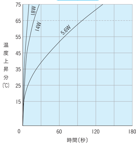
温度上昇特性
