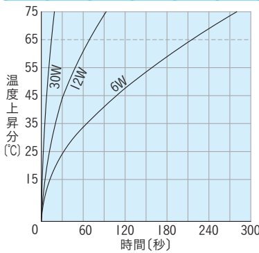
温度上昇特性 CA-134804 / CA-134807
