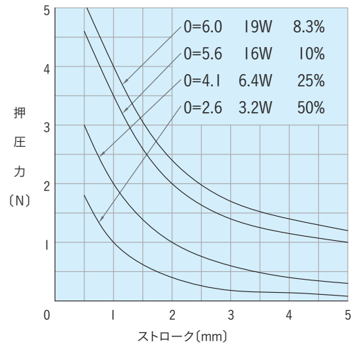
吸引力特性
