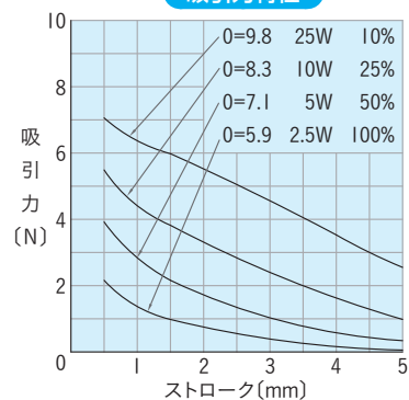
標準コイル表
