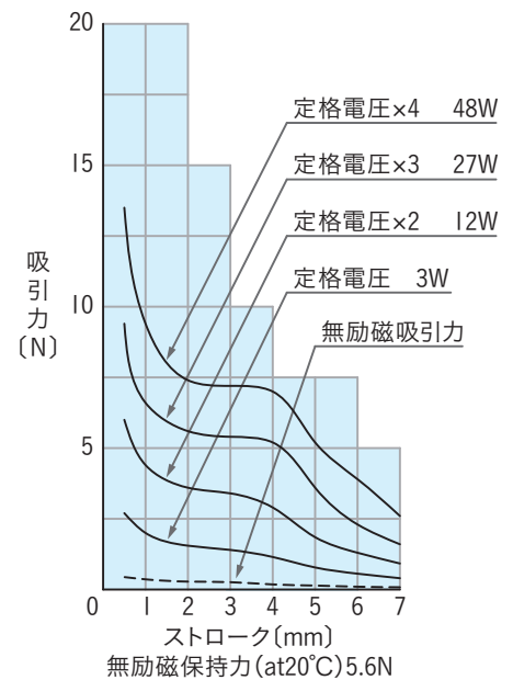
吸引力特性
