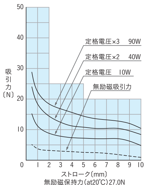
吸引力特性
