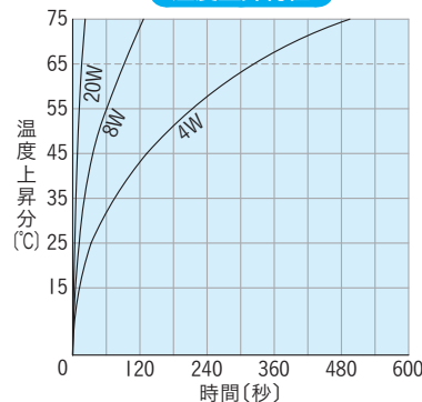
温度上昇特性
