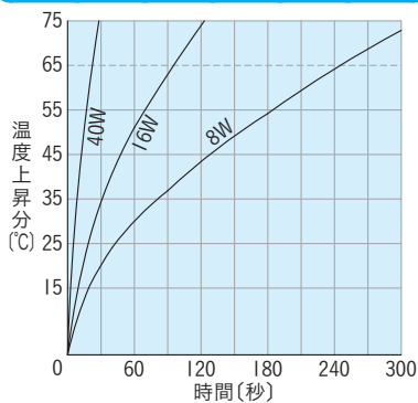
温度上昇特性 CA-174704/CA-174709
