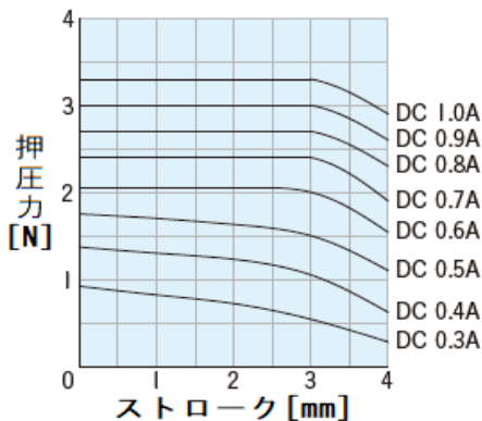
押圧力特性 CA134804
