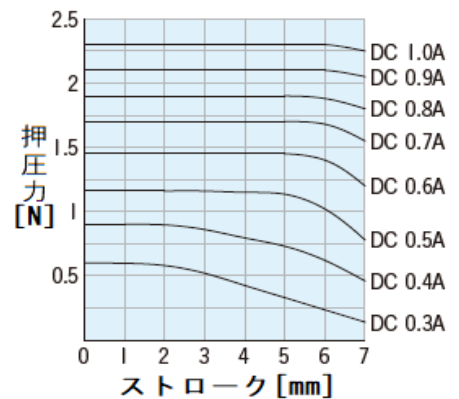
押圧力特性 CA134807
