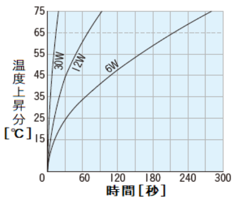
温度上昇特性 (CA134804/134807)
