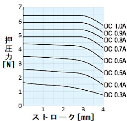
押圧力特性 CA174704
