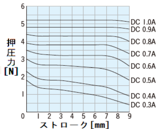
押圧力特性 CA174709
