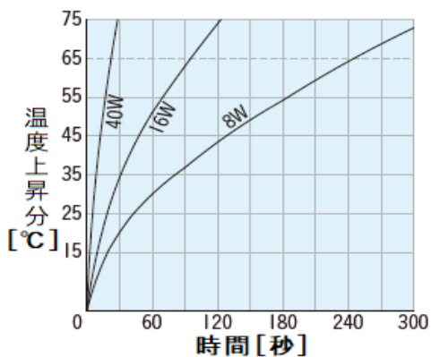
温度上昇特性 (CA174704/174709)
